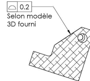
COUPE J-J
