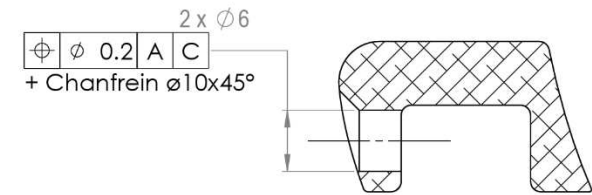
COUPE K-K
