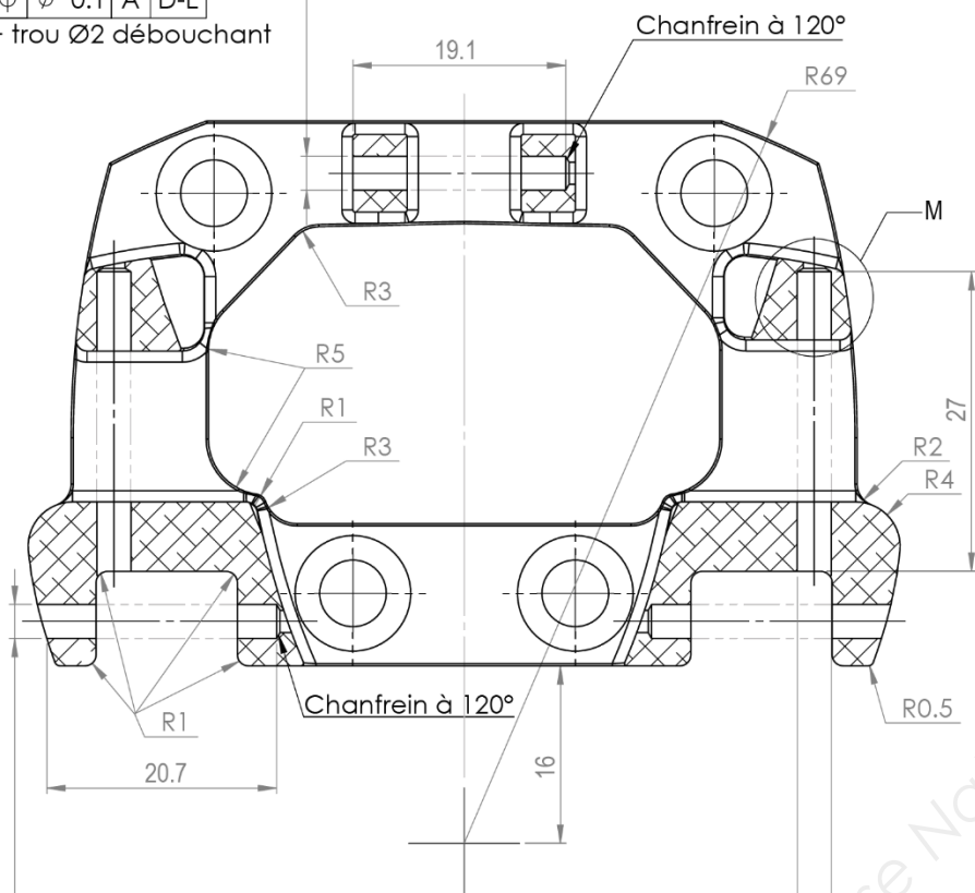
COUPE H-H
